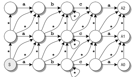
図 18: 誤字 / 脱字を許容する状態遷移機械
